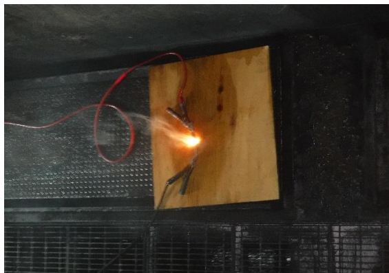
ショートによる火災の再現
